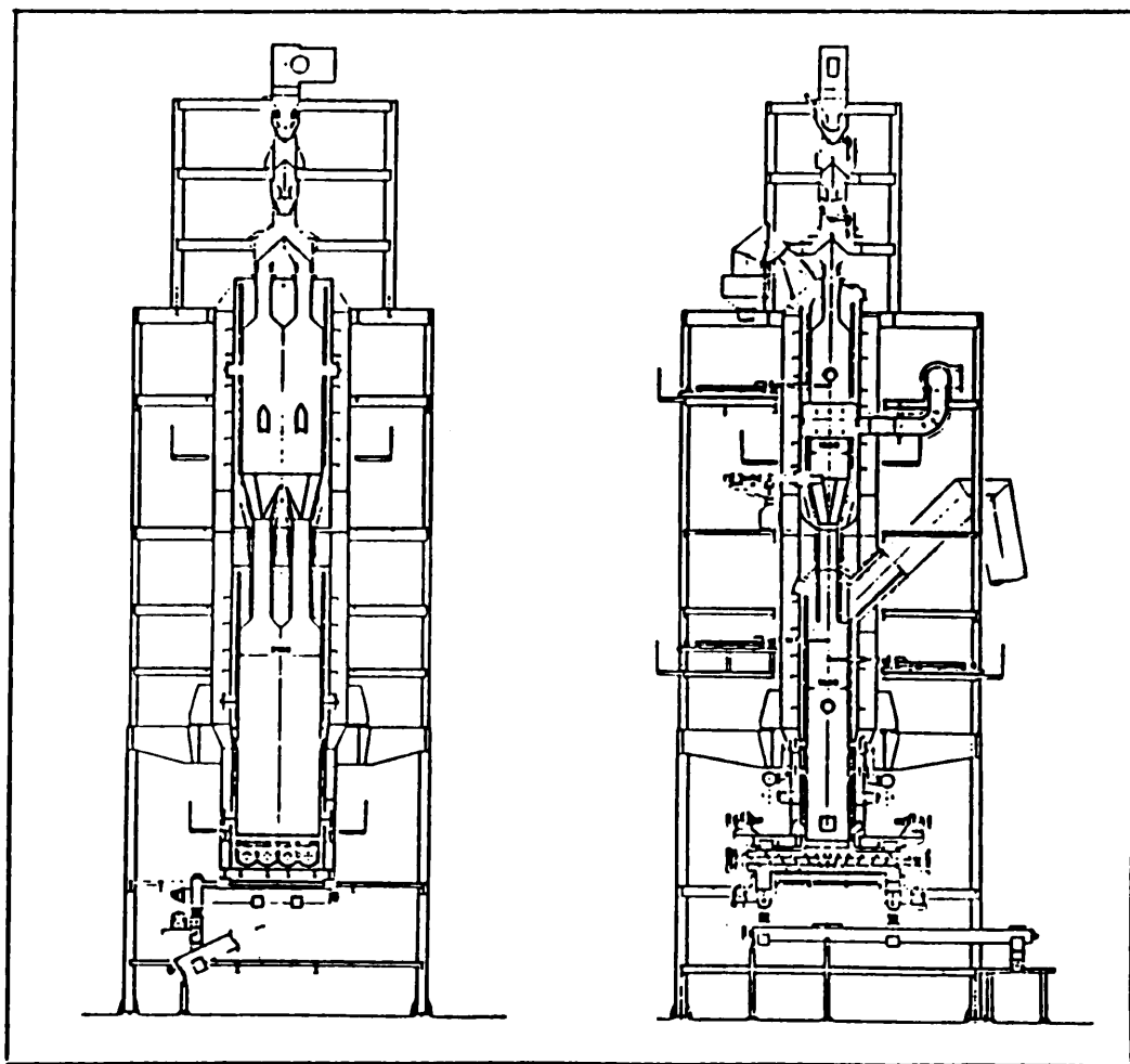
Fig. 4 Shaft type retort
